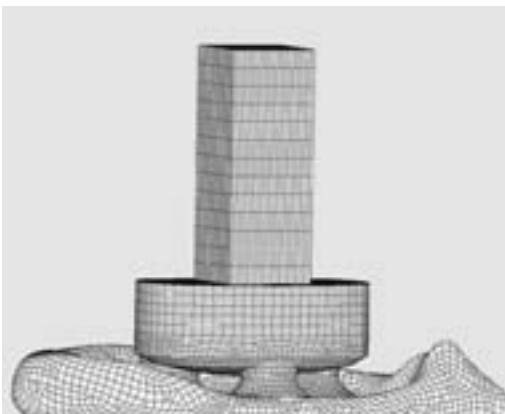
Abb. 1: FE-Modell des Prothesenschuhs auf der Steigbügelfußplatte. Die drei Halbkugeln auf der Unterseite des Prothesenschuhs sind hier zu 60 % ihrer Oberfläche (104 \mu\text{m} Höhe) in neu gebildetes Gewebe eingebettet.
