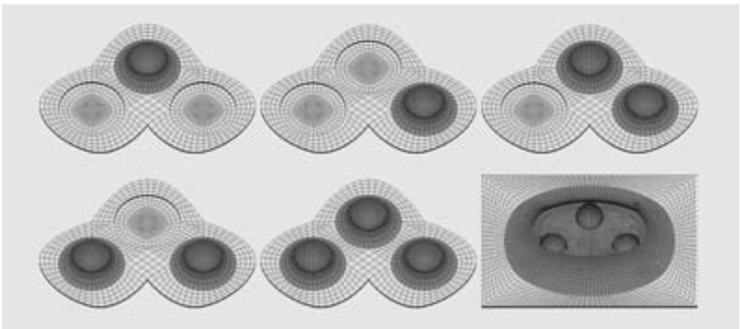
Abb. 2: Mögliche Kombinationen der Einbettung des Prothesenschuhs auf der Steigbügelfußplatte. Neben der Einbettung von jeweils einer bzw. zwei Halbkugeln wurde das Szenario eines vollständig von neu gebildetem Gewebe umschlossenen Prothesenschuhs simuliert.
